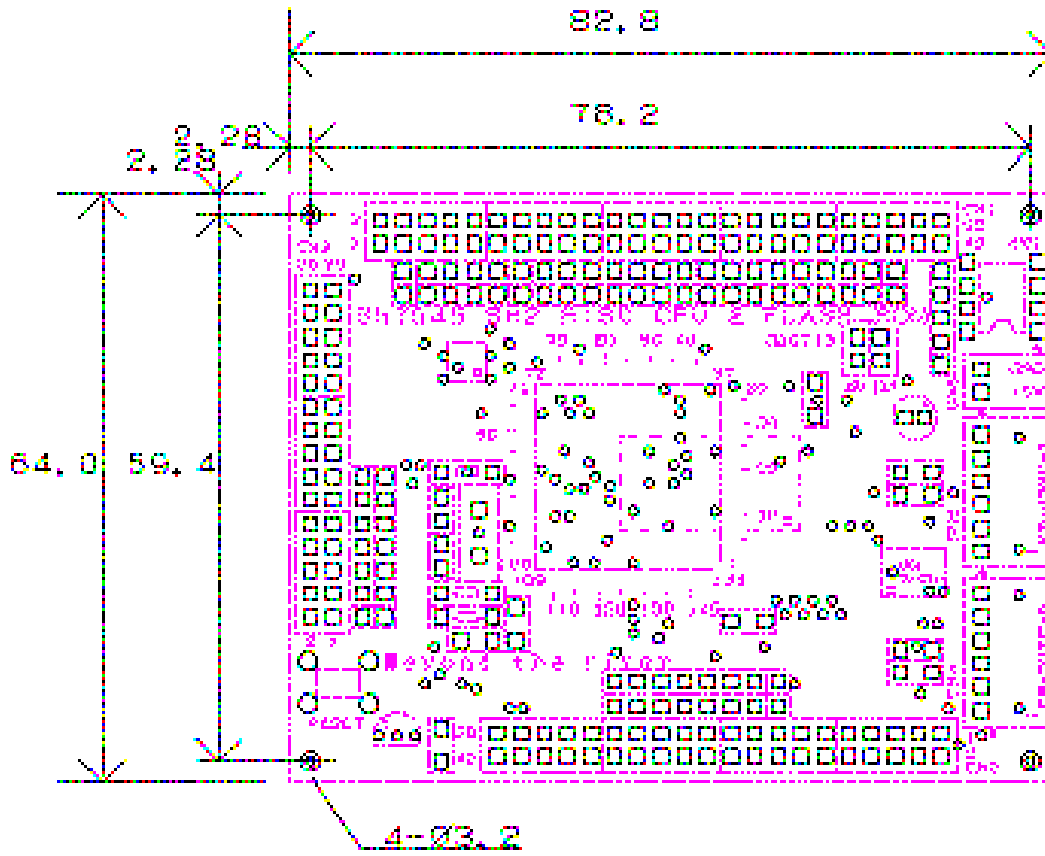
SH7045外形封込図
